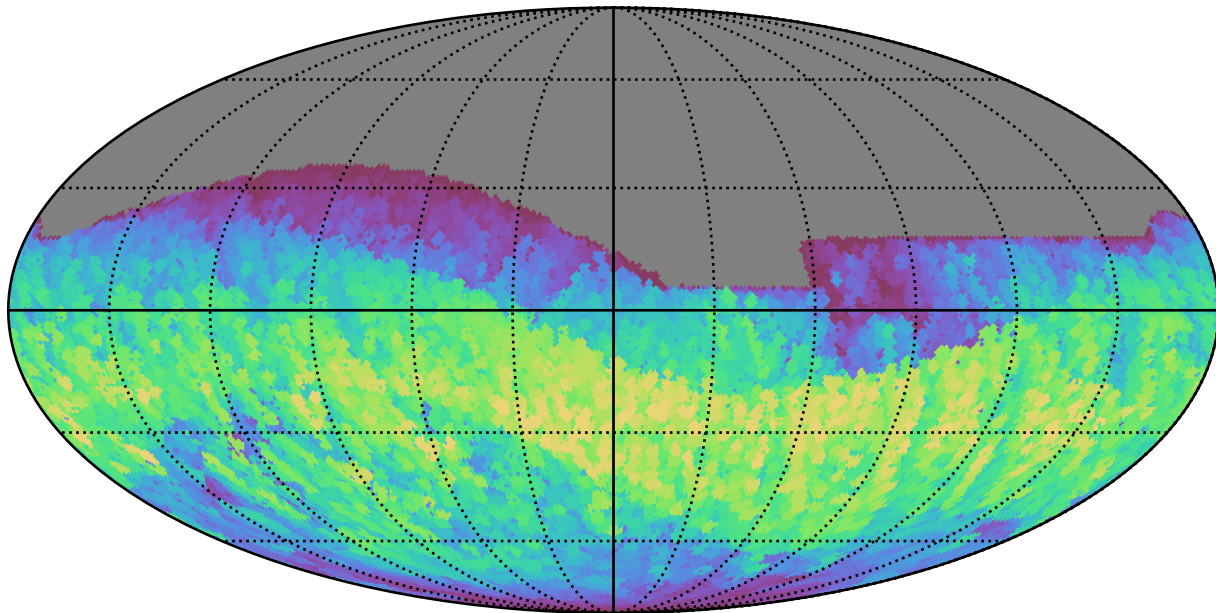
weather_cloudso6v3.4_10yrs All sky z band: Max normairmass
