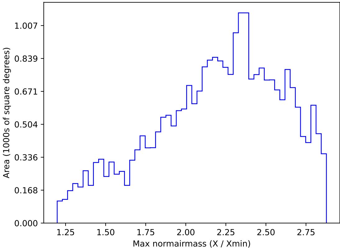
weather_cloudso6v3.4_10yrs All sky z band: Max normairmass
