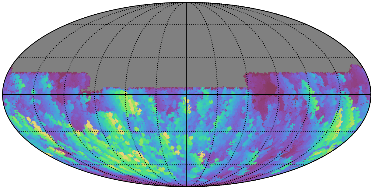
weather_cloudso6v3.4_10yrs All sky u band: Max normairmass
