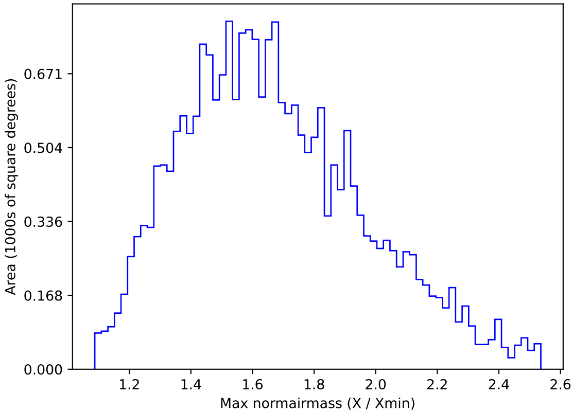
weather_cloudso6v3.4_10yrs All sky u band: Max normairmass
