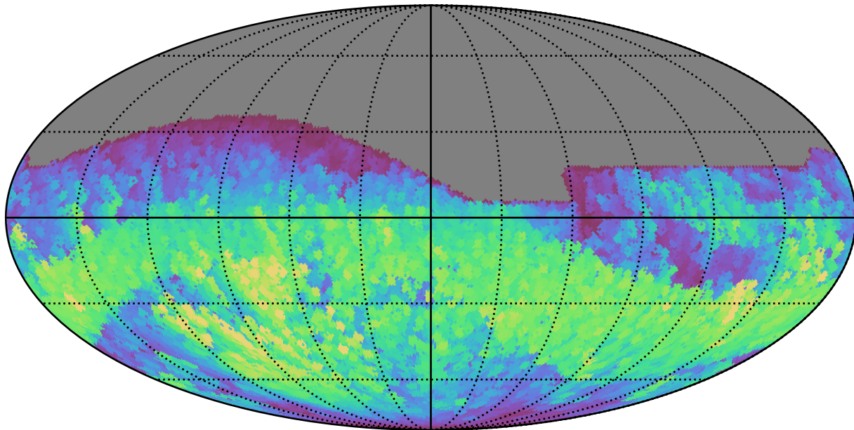
weather_cloudso6v3.4_10yrs All sky r band: Max normairmass
