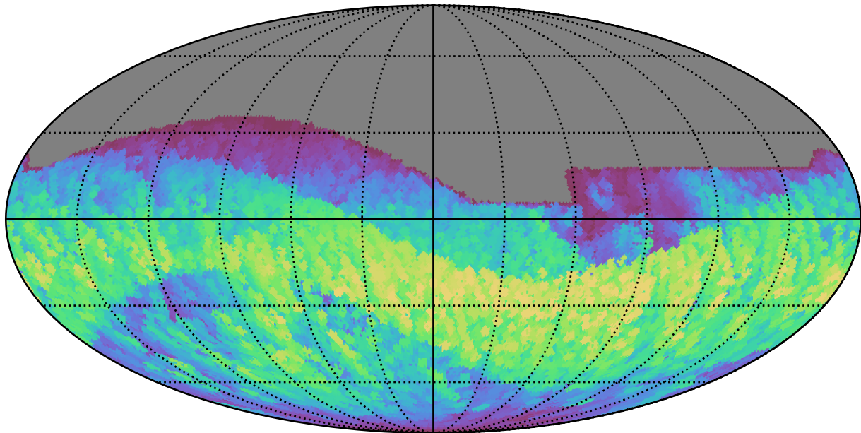
weather_cloudso6v3.4_10yrs All sky i band: Max normairmass
