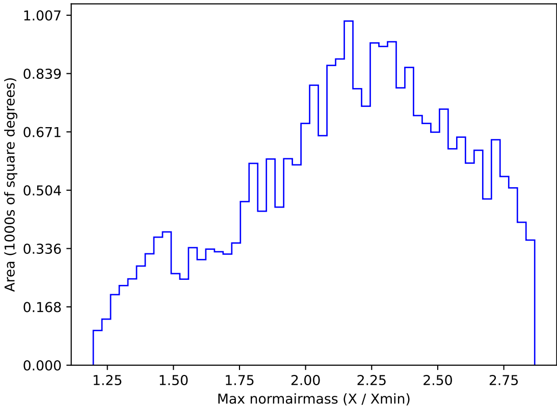
weather_cloudso6v3.4_10yrs All sky i band: Max normairmass
