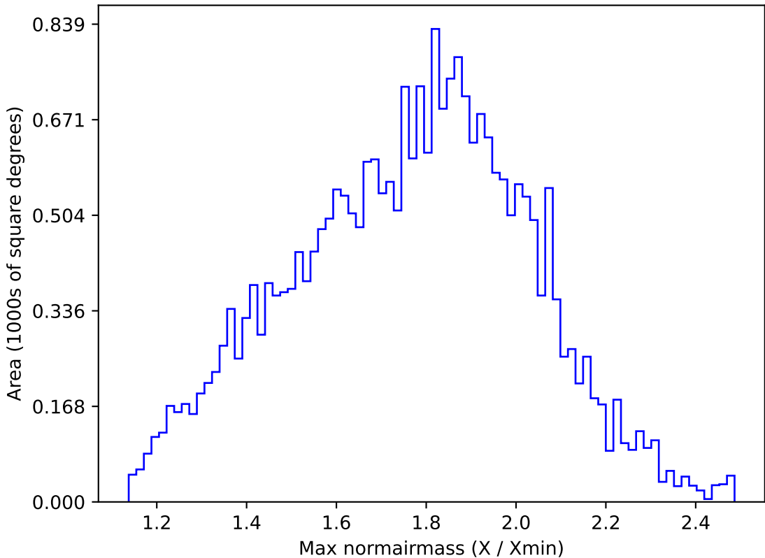
weather_cloudso6v3.4_10yrs All sky g band: Max normairmass
