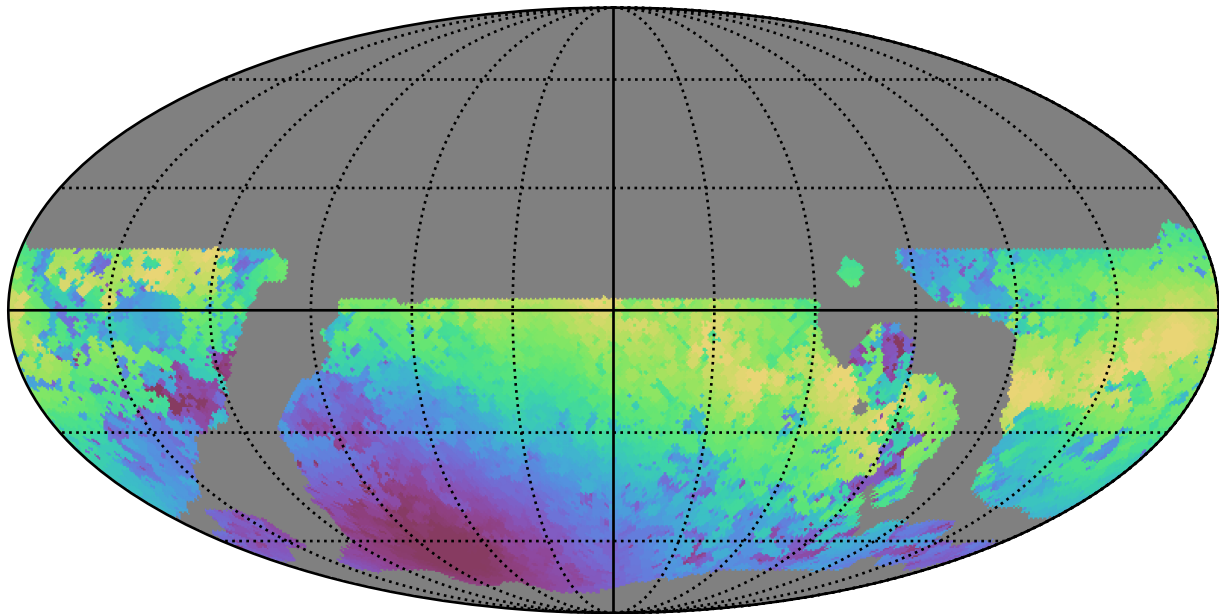
weather_cloudso6v3.4_10yrs WFD y band: Max moonDistance
