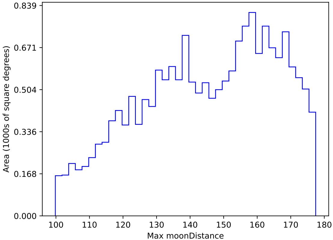
weather_cloudso6v3.4_10yrs WFD y band: Max moonDistance
