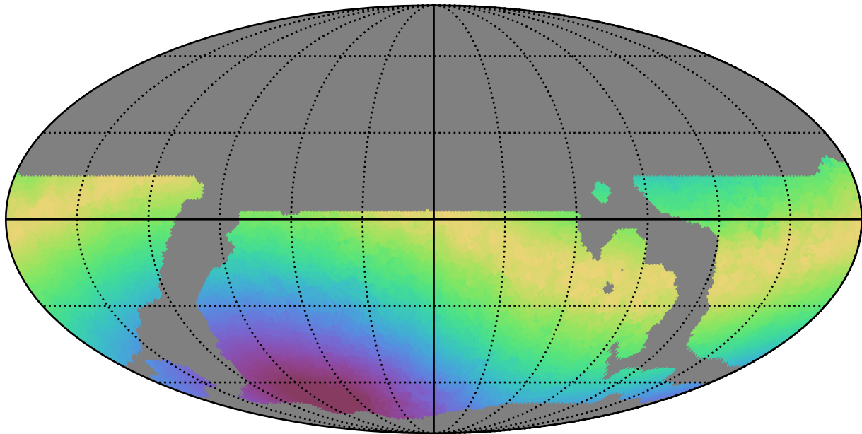
weather_cloudso6v3.4_10yrs WFD i band: Max moonDistance
