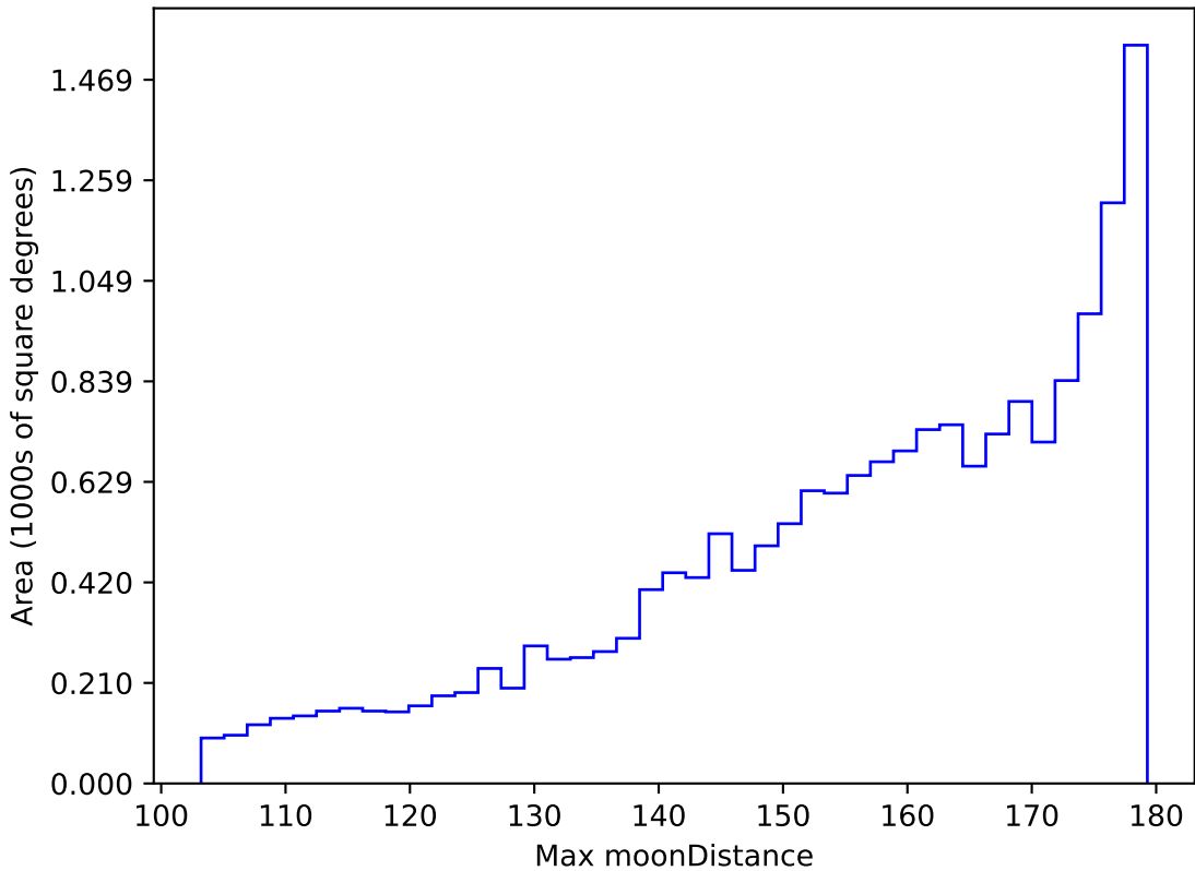
weather_cloudso6v3.4_10yrs WFD i band: Max moonDistance
