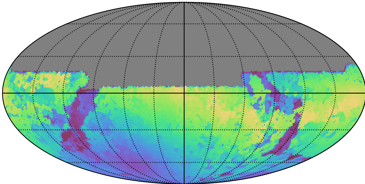
weather_cloudso6v3.4_10yrs All sky y band: Max moonDistance
