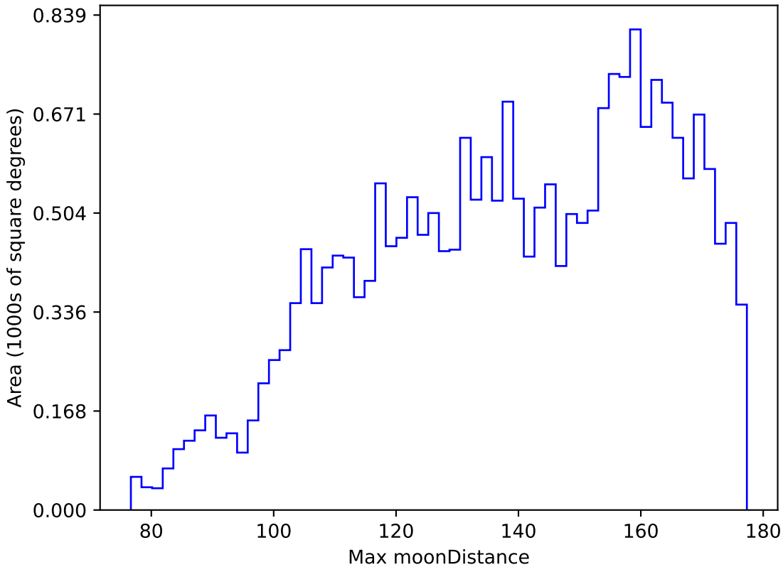
weather_cloudso6v3.4_10yrs All sky y band: Max moonDistance
