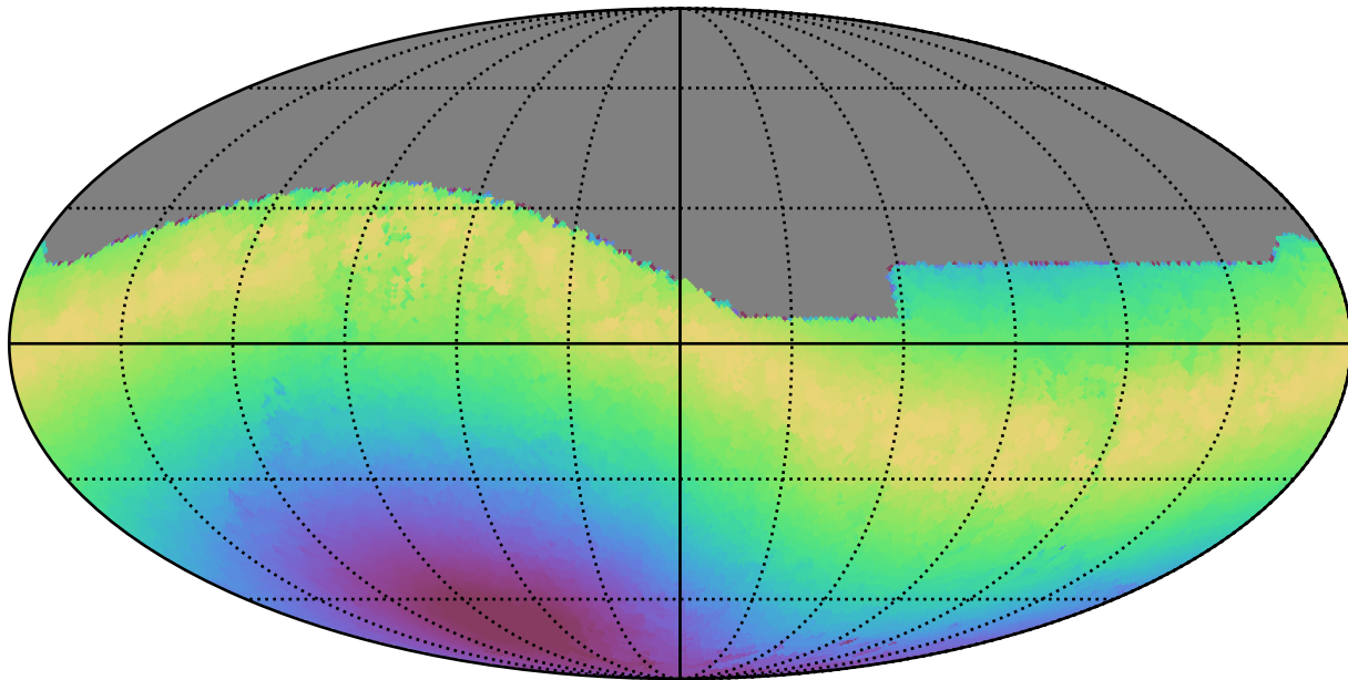
weather_cloudso6v3.4_10yrs All sky i band: Max moonDistance
