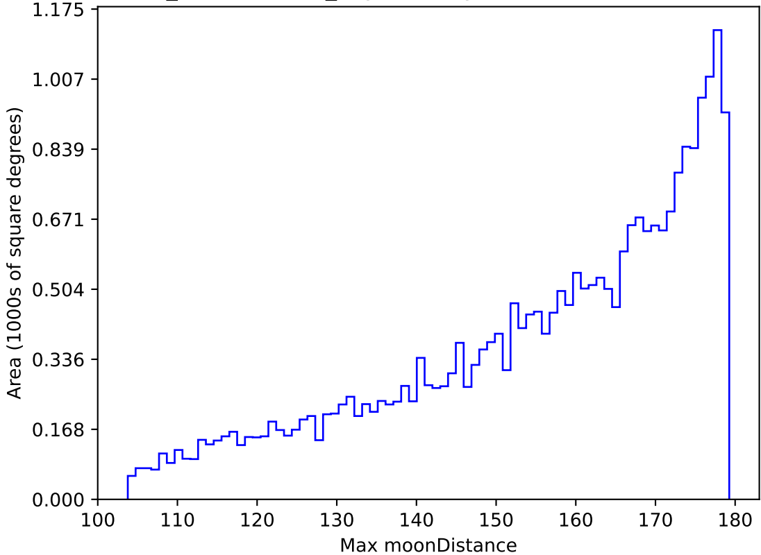
weather_cloudso6v3.4_10yrs All sky i band: Max moonDistance
