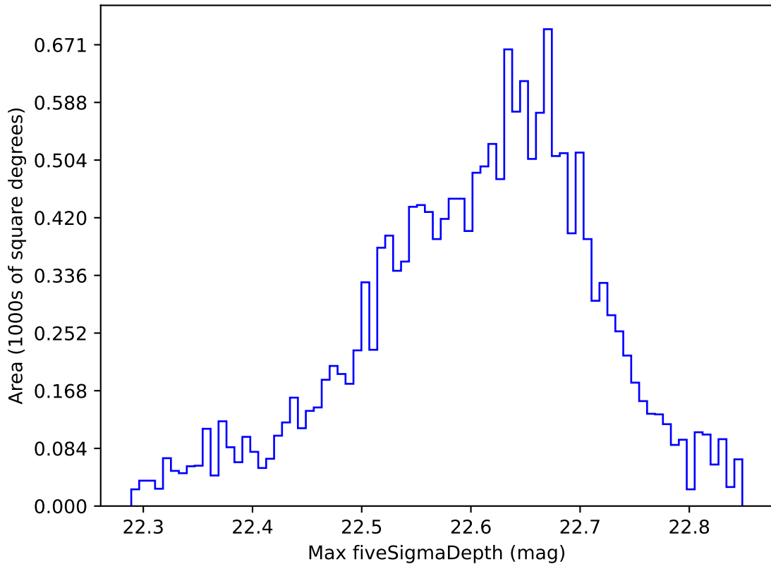
weather_cloudso6v3.4_10yrs WFD y band: Max fiveSigmaDepth
