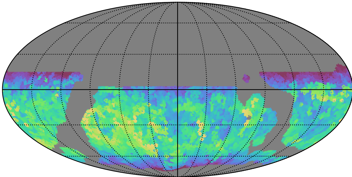
weather_cloudso6v3.4_10yrs WFD i band: Max fiveSigmaDepth
