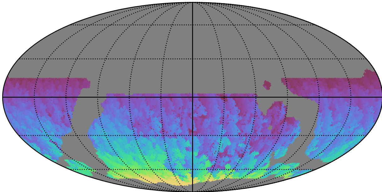
weather_cloudso6v3.4_10yrs WFD y band: Max HA
