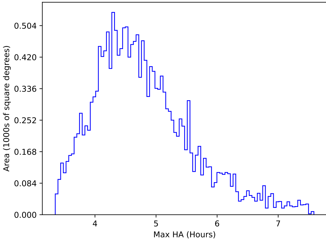
weather_cloudso6v3.4_10yrs WFD y band: Max HA
