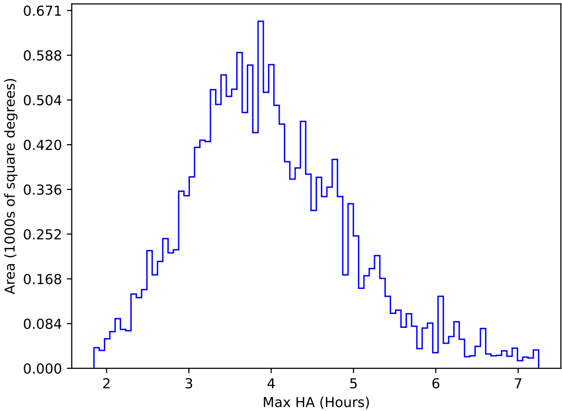
weather_cloudso6v3.4_10yrs WFD u band: Max HA
