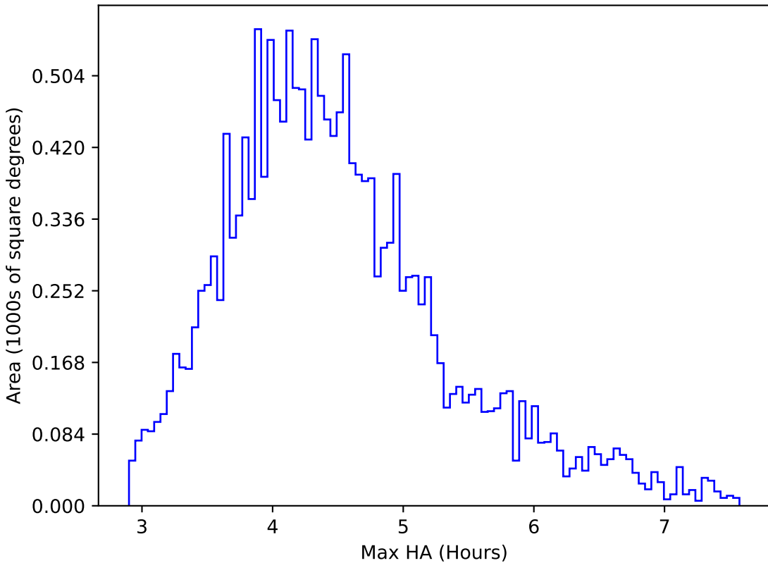
weather_cloudso6v3.4_10yrs WFD r band: Max HA
