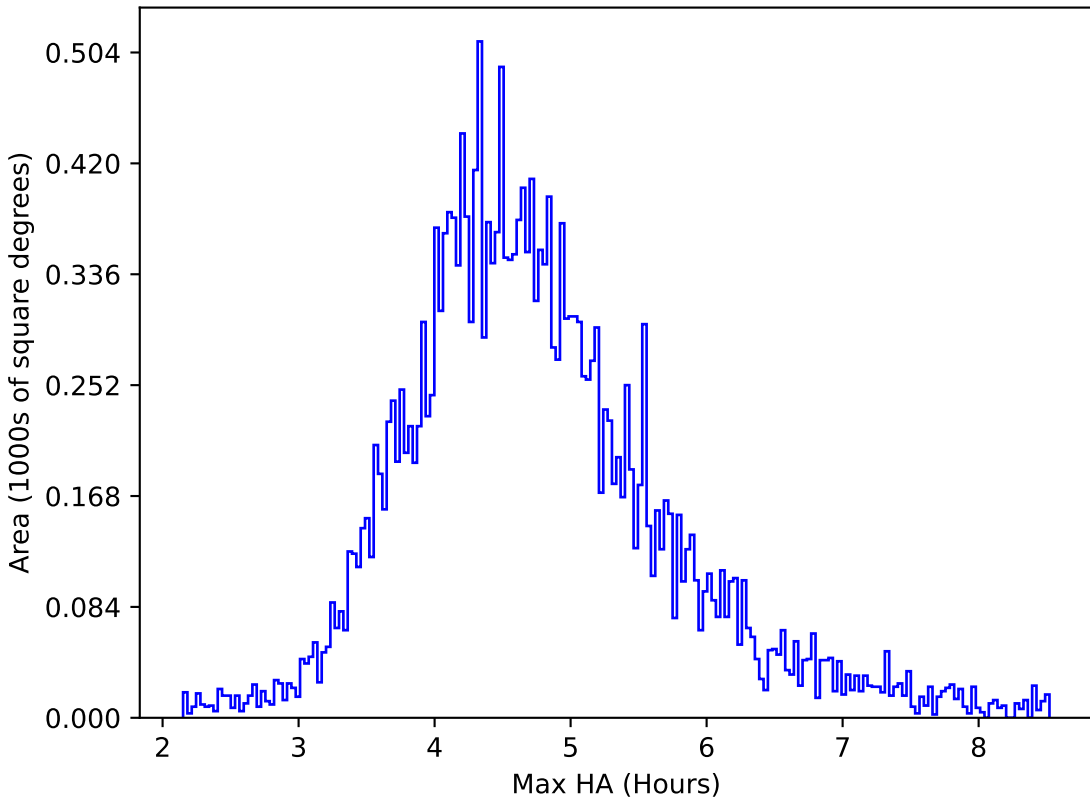
weather_cloudso6v3.4_10yrs All sky y band: Max HA
