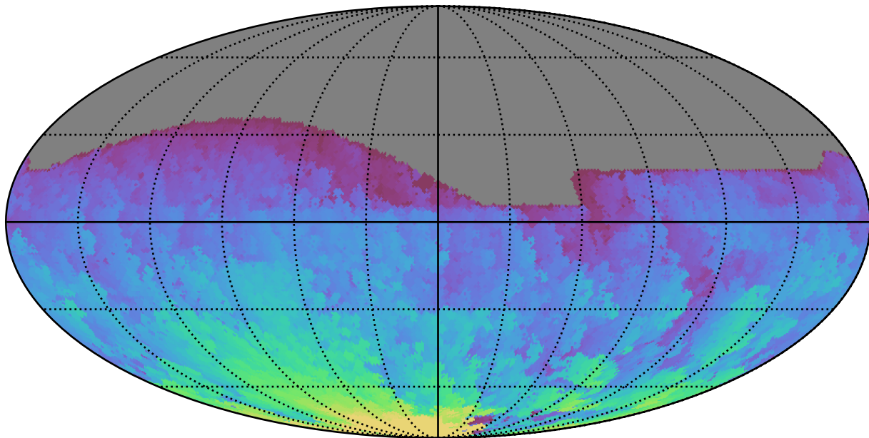
weather_cloudso6v3.4_10yrs All sky r band: Max HA
