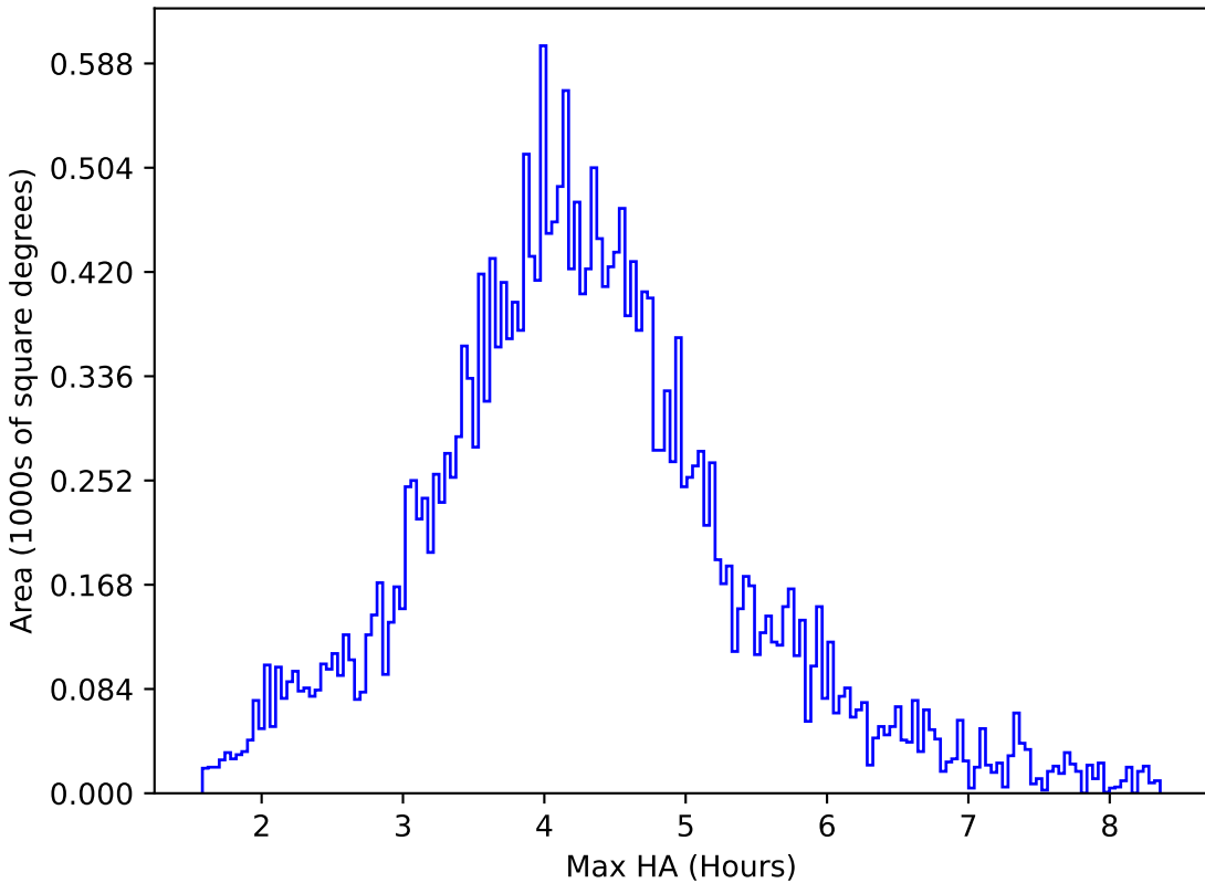
weather_cloudso6v3.4_10yrs All sky r band: Max HA
