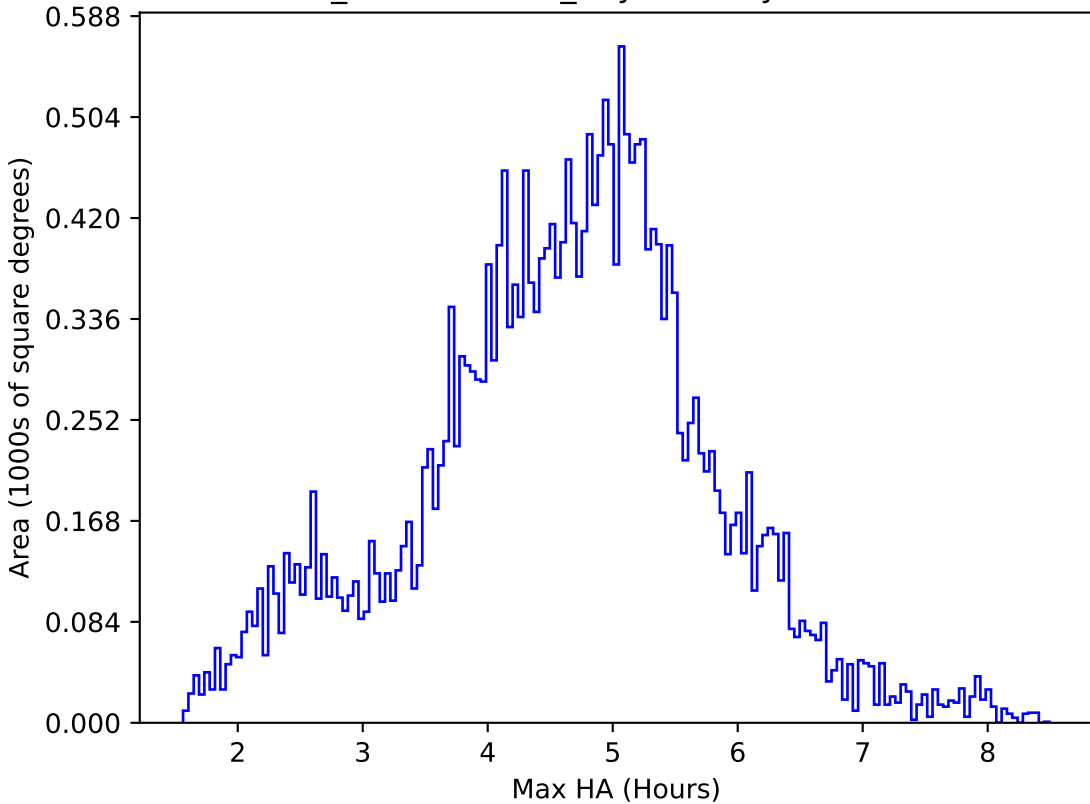
weather_cloudso6v3.4_10yrs All sky i band: Max HA
