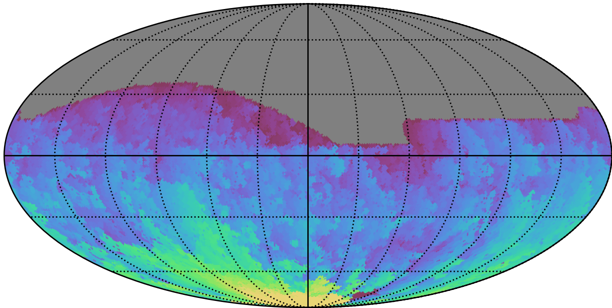
weather_cloudso6v3.4_10yrs All sky g band: Max HA
