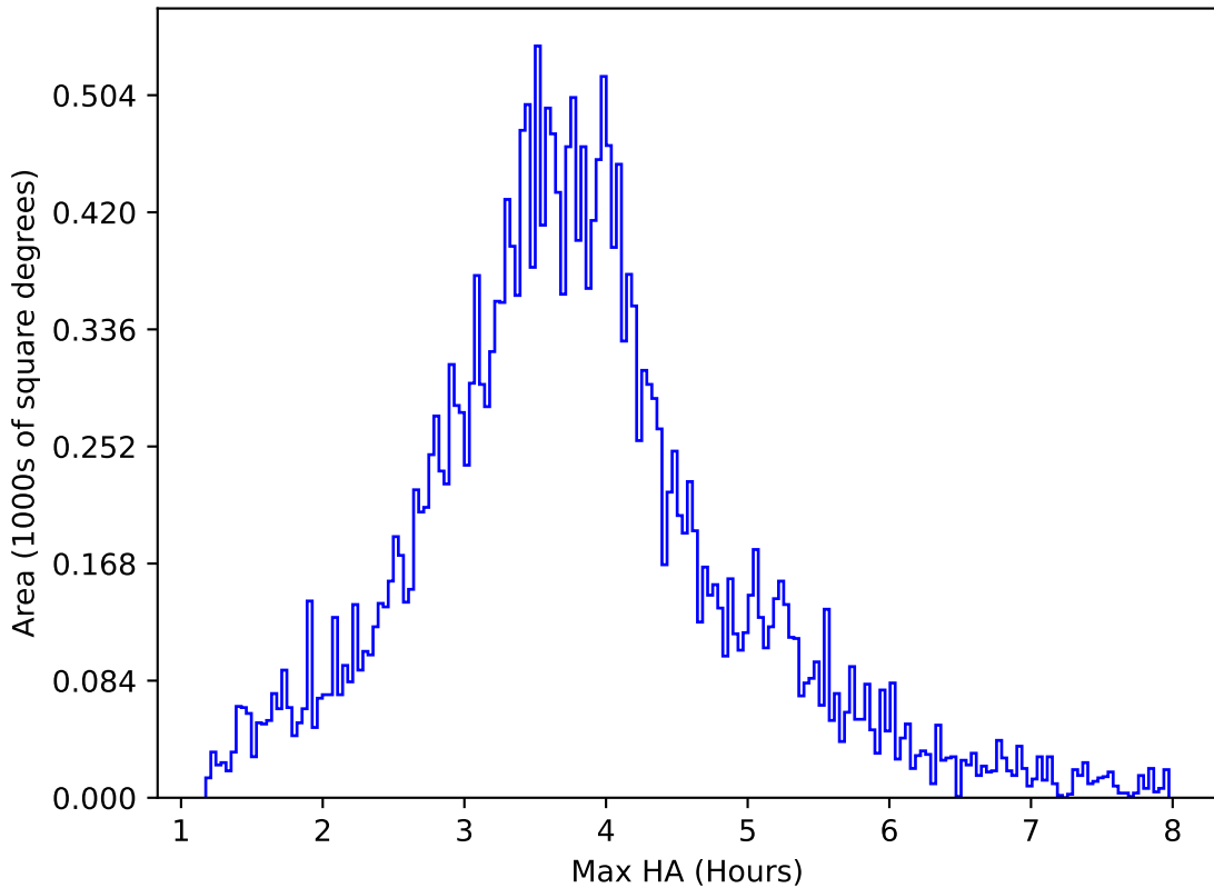
weather_cloudso6v3.4_10yrs All sky g band: Max HA
