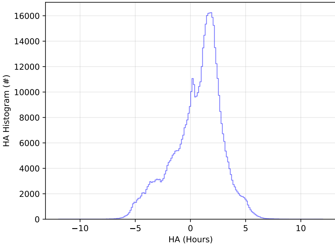
weather_cloudso6v3.4_10yrs WFD i band: HA Histogram
