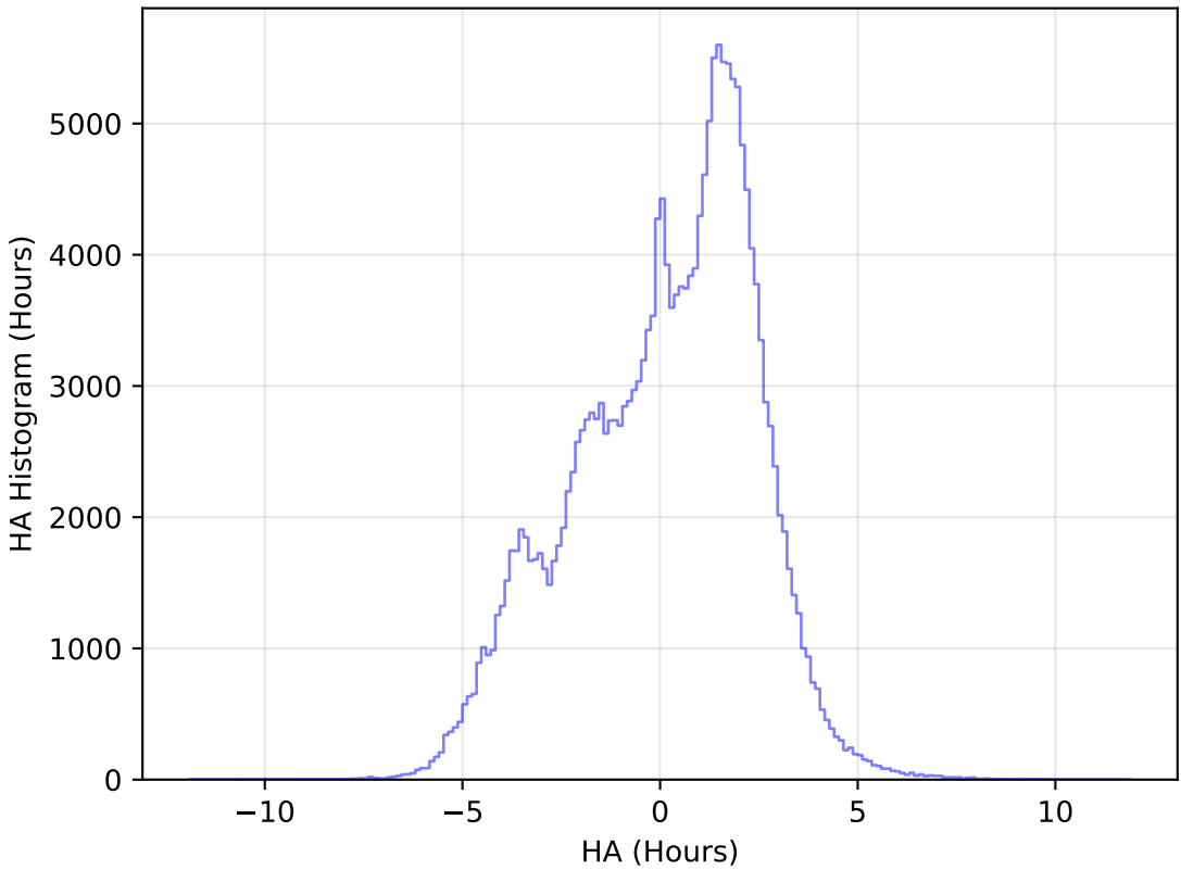
weather_cloudso6v3.4_10yrs WFD g band: HA Histogram
