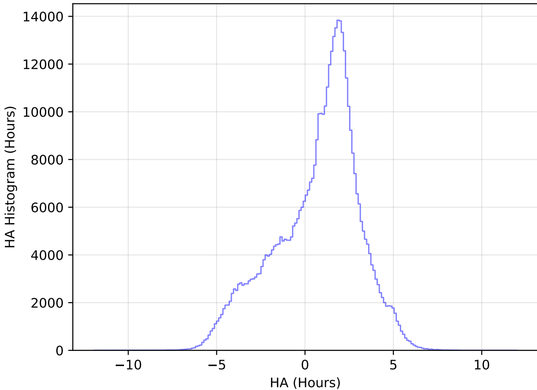
weather_cloudso6v3.4_10yrs All sky z band: HA Histogram
