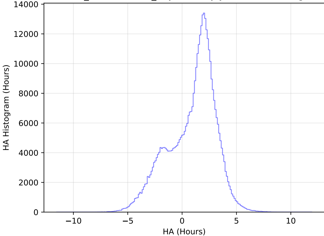
weather_cloudso6v3.4_10yrs All sky y band: HA Histogram
