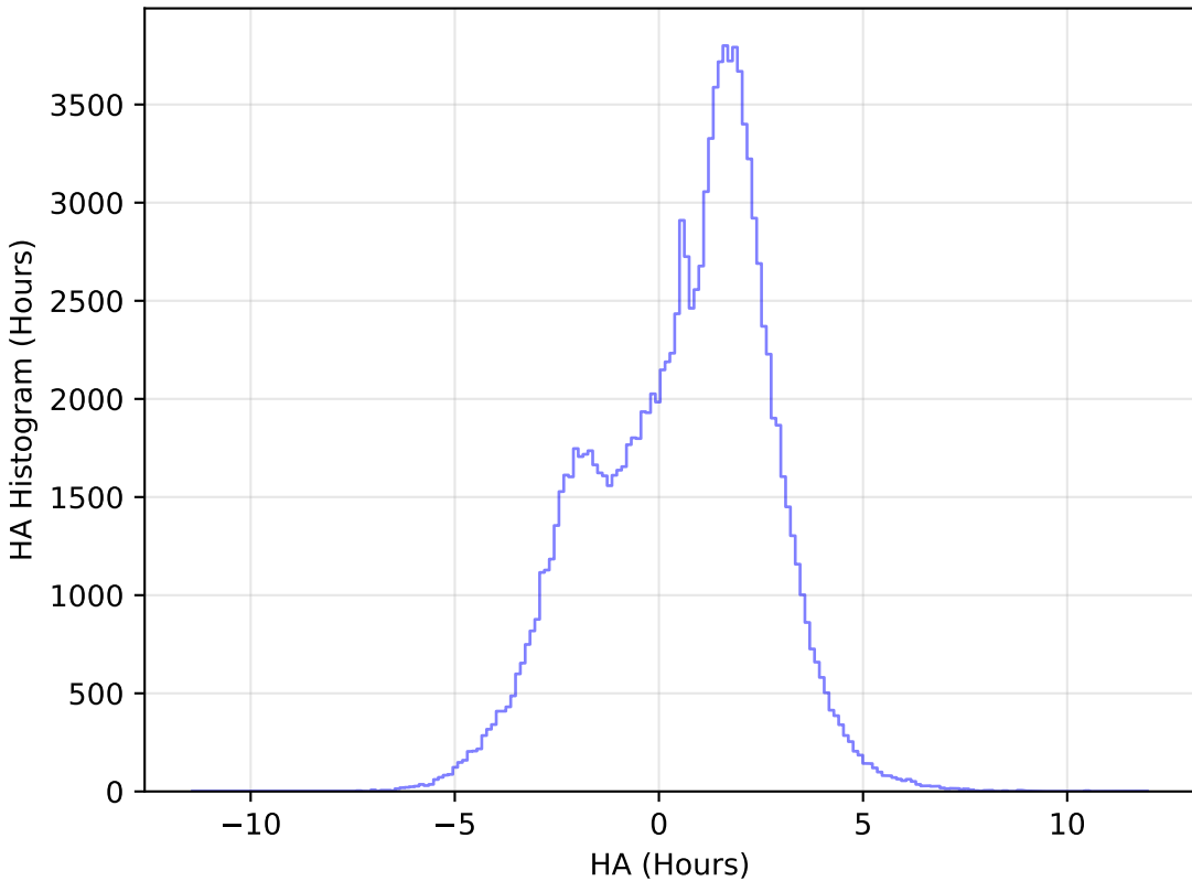
weather_cloudso6v3.4_10yrs All sky u band: HA Histogram
