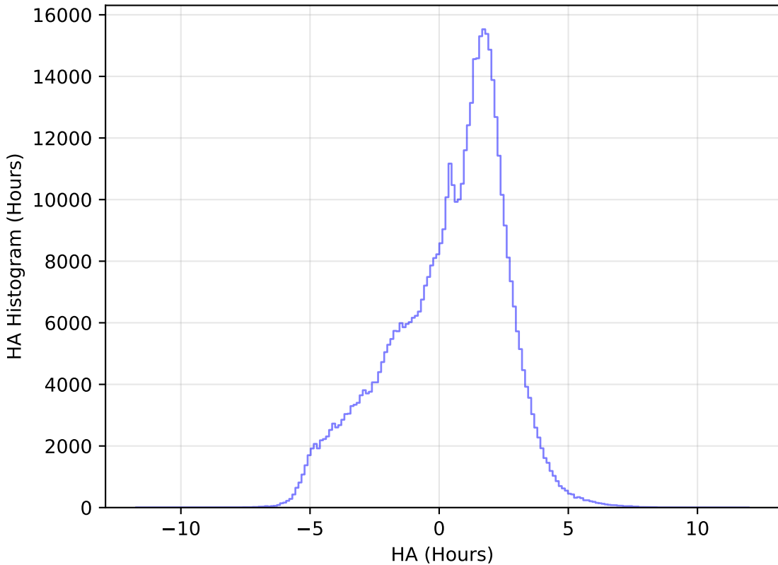
weather_cloudso6v3.4_10yrs All sky r band: HA Histogram
