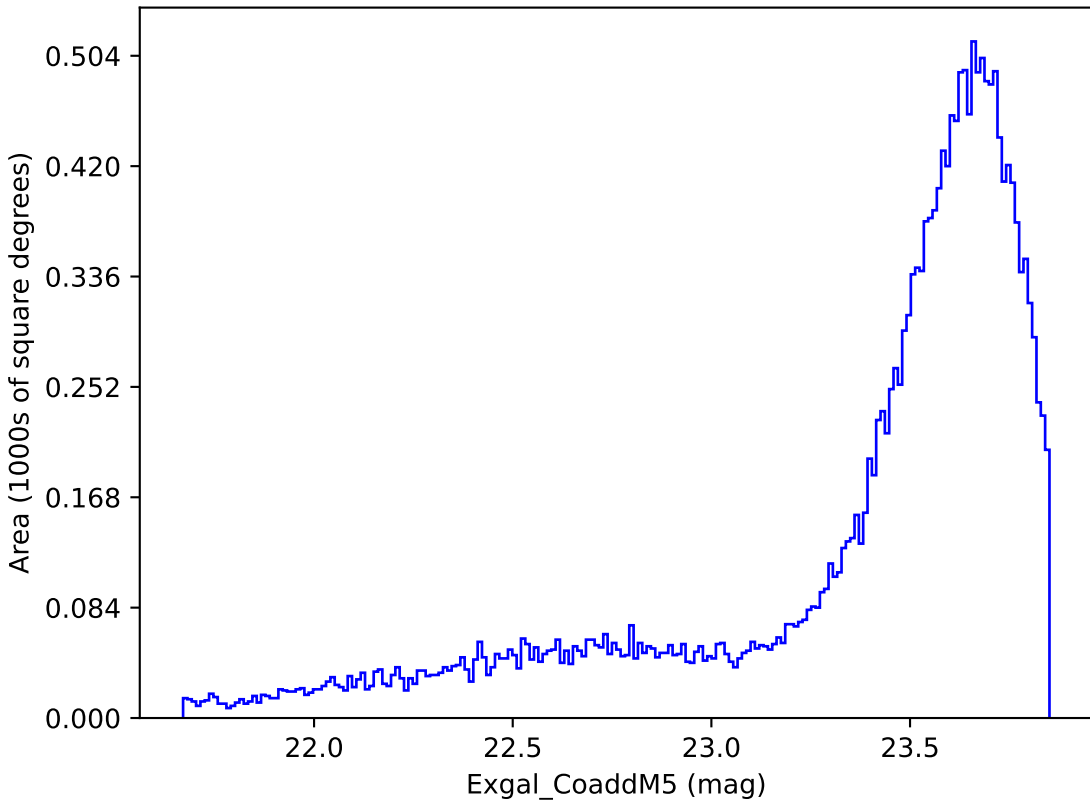
weather_cloudso6v3.4_10yrs Yr 1 y band: Exgal_CoaddM5
