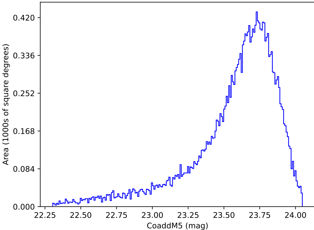
weather_cloudso6v3.4_10yrs Yr 1 y band: CoaddM5
