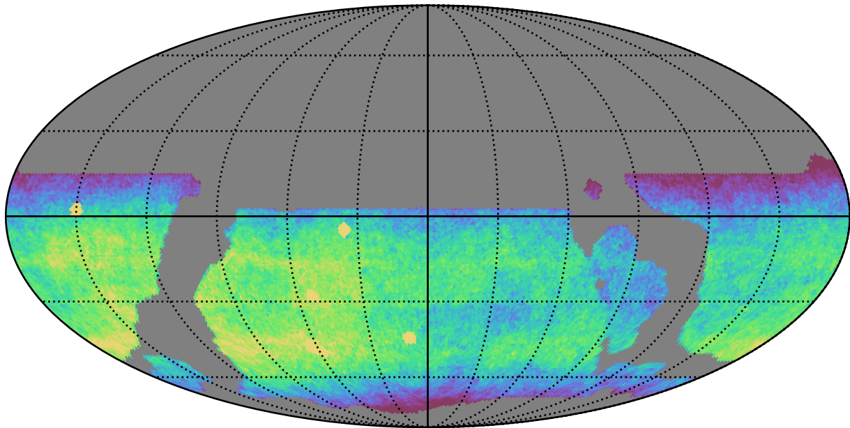
weather_cloudso6v3.4_10yrs WFD z band: CoaddM5
