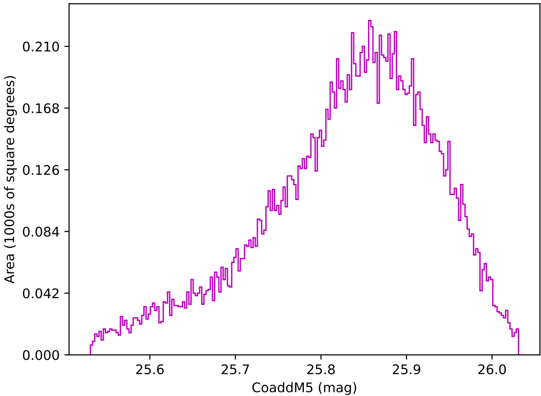
weather_cloudso6v3.4_10yrs WFD z band: CoaddM5
