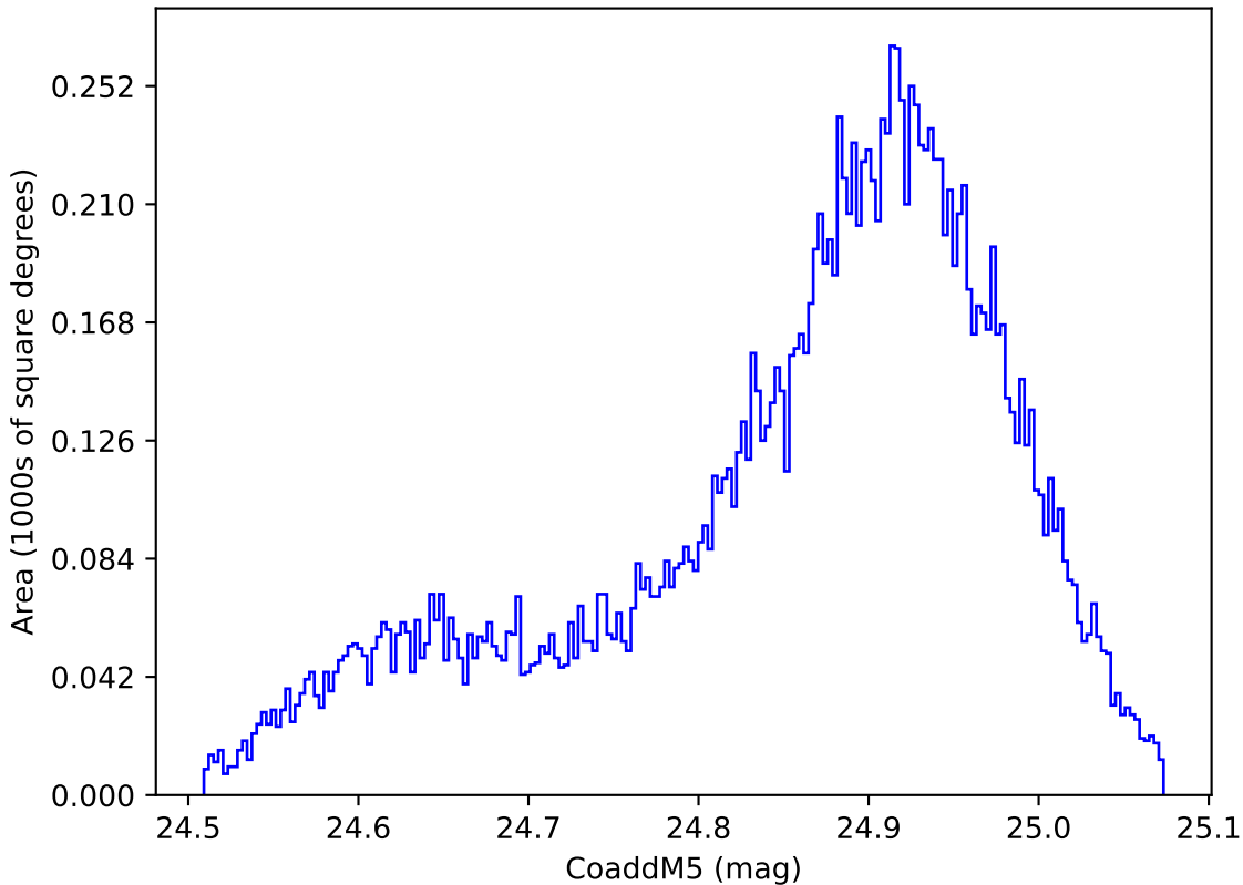
weather_cloudso6v3.4_10yrs WFD y band: CoaddM5
