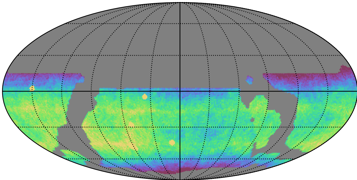
weather_cloudso6v3.4_10yrs WFD i band: CoaddM5
