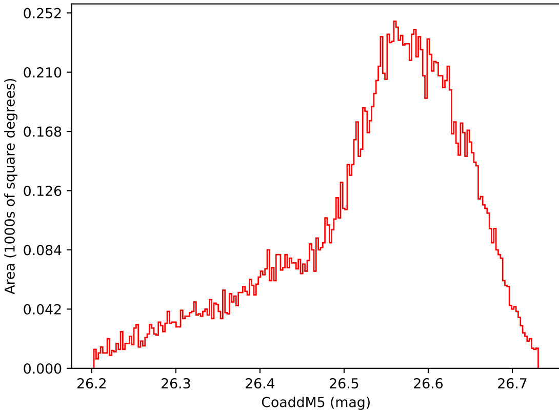
weather_cloudso6v3.4_10yrs WFD i band: CoaddM5
