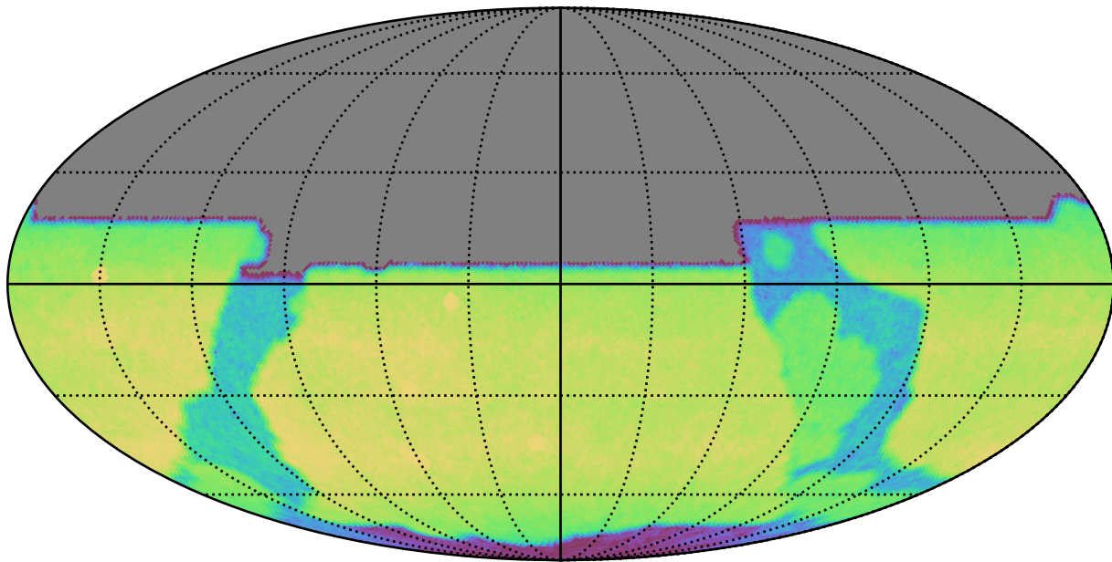
weather_cloudso6v3.4_10yrs All sky y band: CoaddM5
