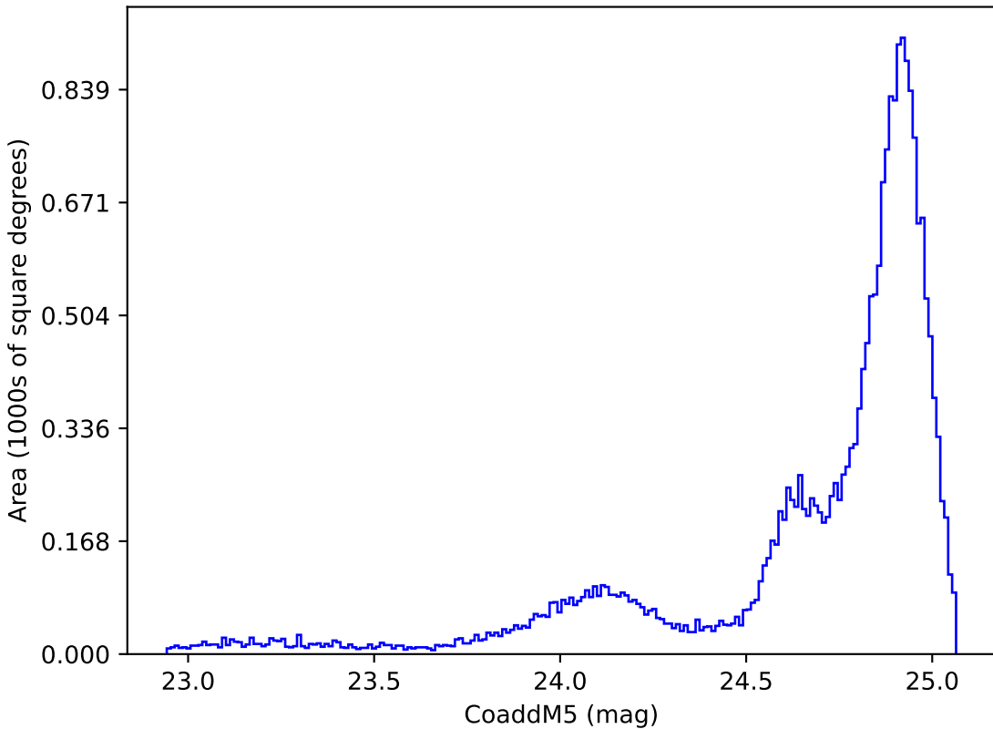
weather_cloudso6v3.4_10yrs All sky y band: CoaddM5
