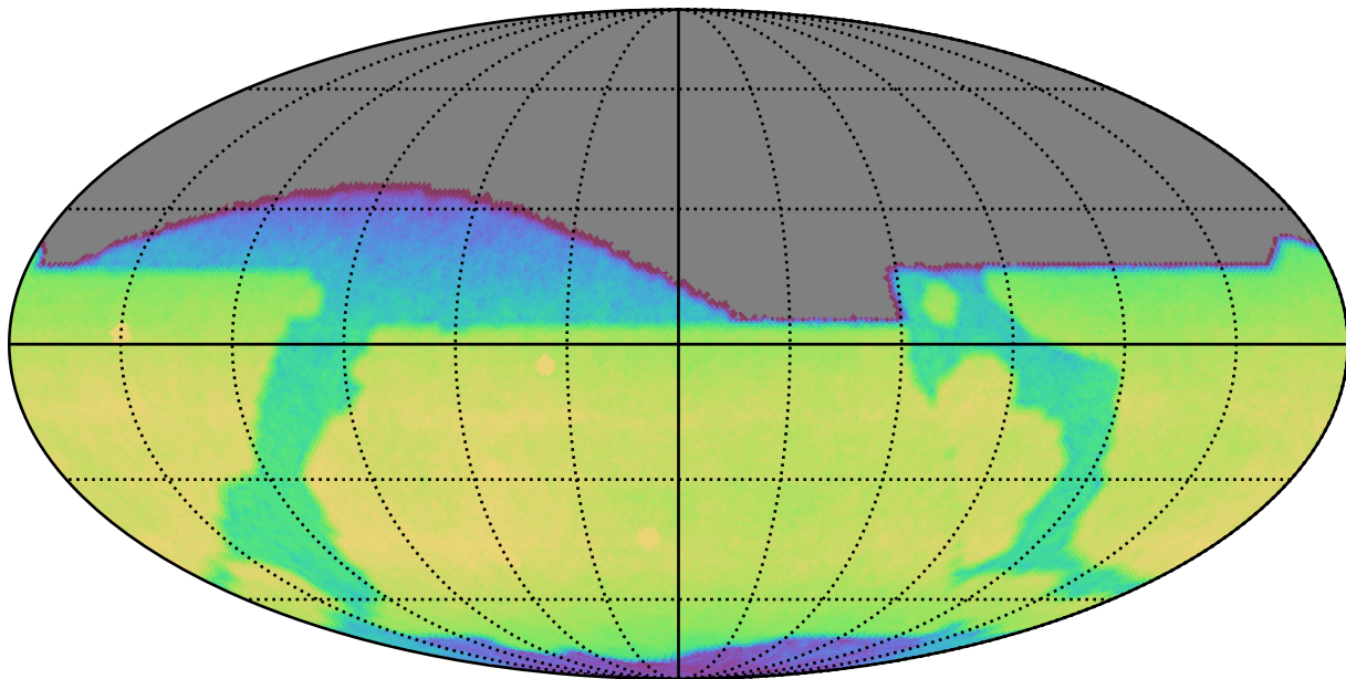
weather_cloudso6v3.4_10yrs All sky i band: CoaddM5
