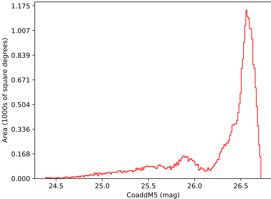
weather_cloudso6v3.4_10yrs All sky i band: CoaddM5
