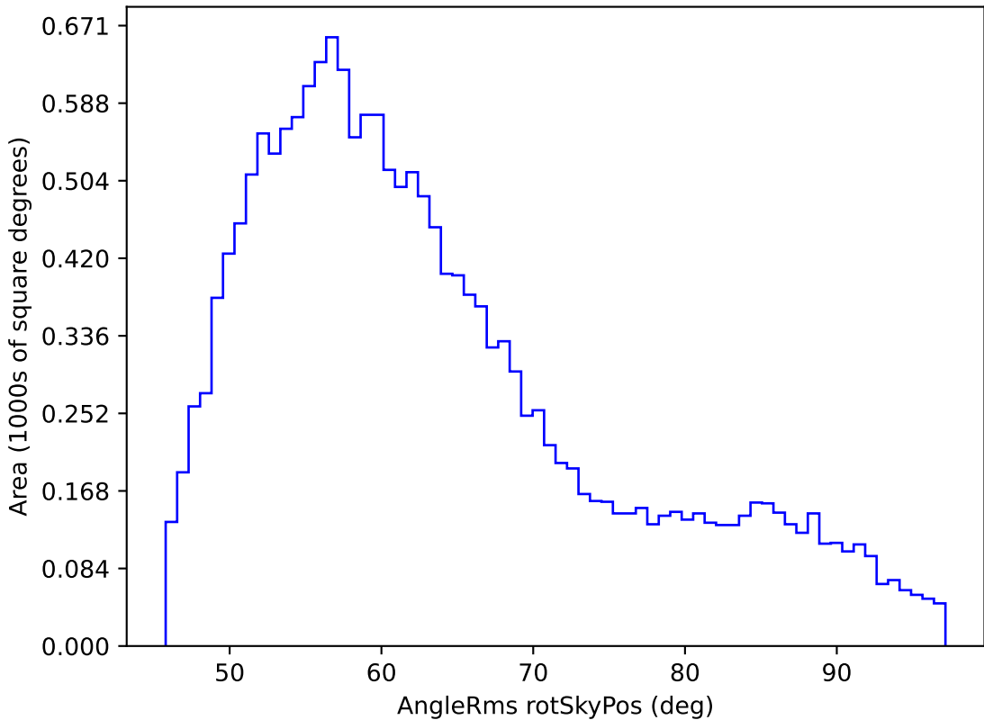
weather_cloudso6v3.4_10yrs WFD y band: AngleRms rotSkyPos
