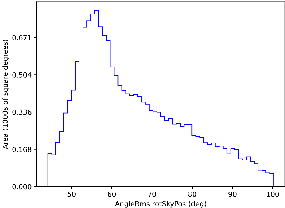
weather_cloudso6v3.4_10yrs WFD u band: AngleRms rotSkyPos
