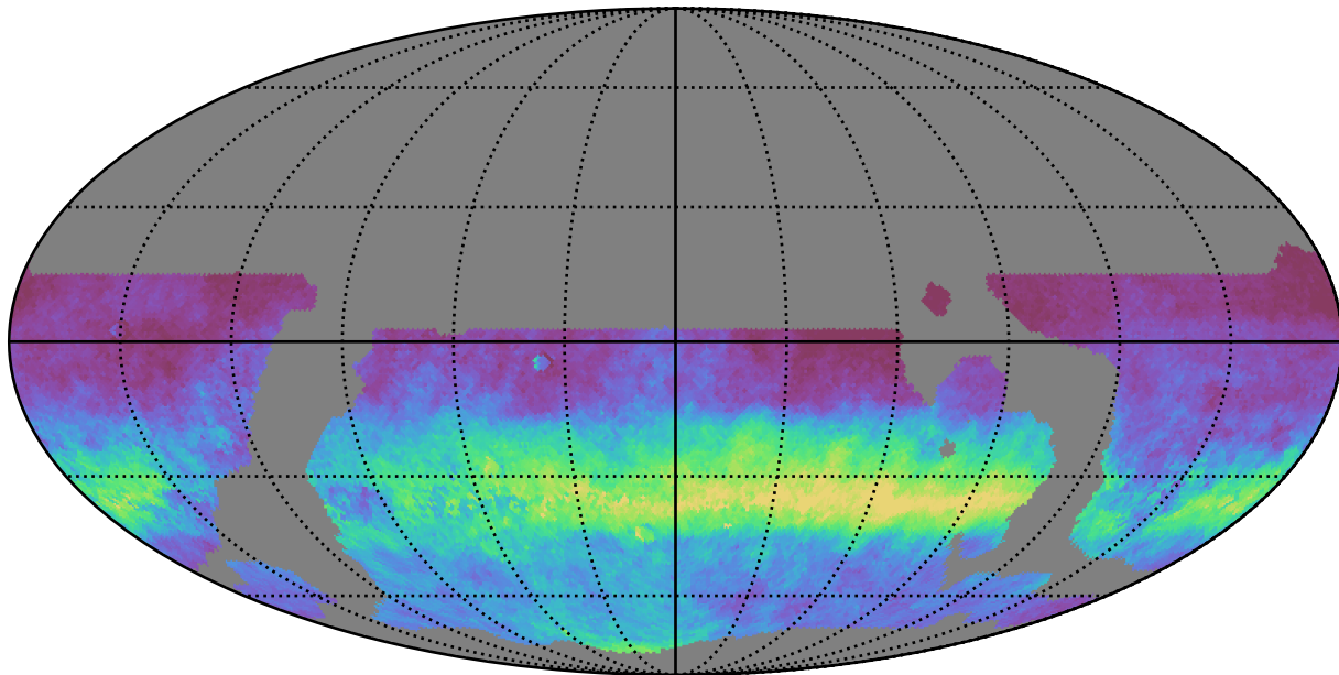
weather_cloudso6v3.4_10yrs WFD r band: AngleRms rotSkyPos
