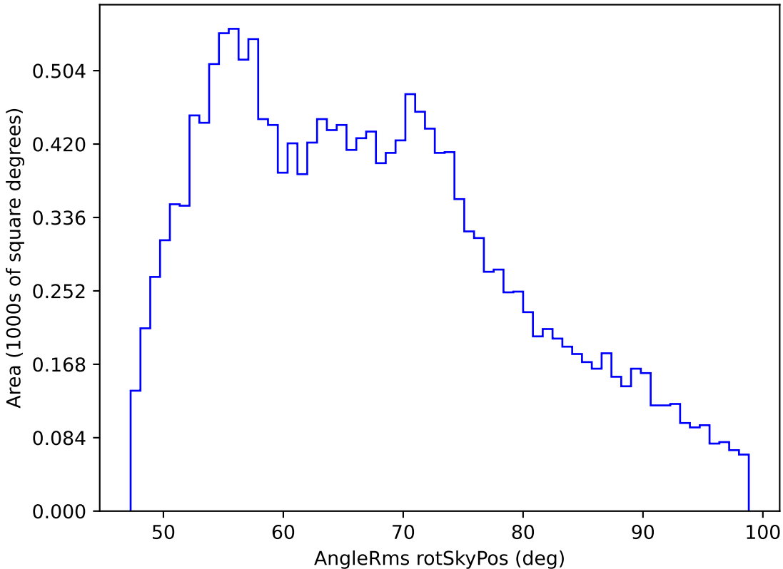
weather_cloudso6v3.4_10yrs WFD r band: AngleRms rotSkyPos
