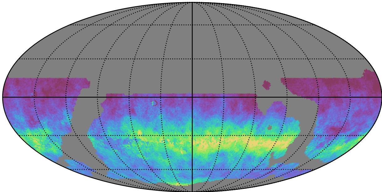
weather_cloudso6v3.4_10yrs WFD i band: AngleRms rotSkyPos
